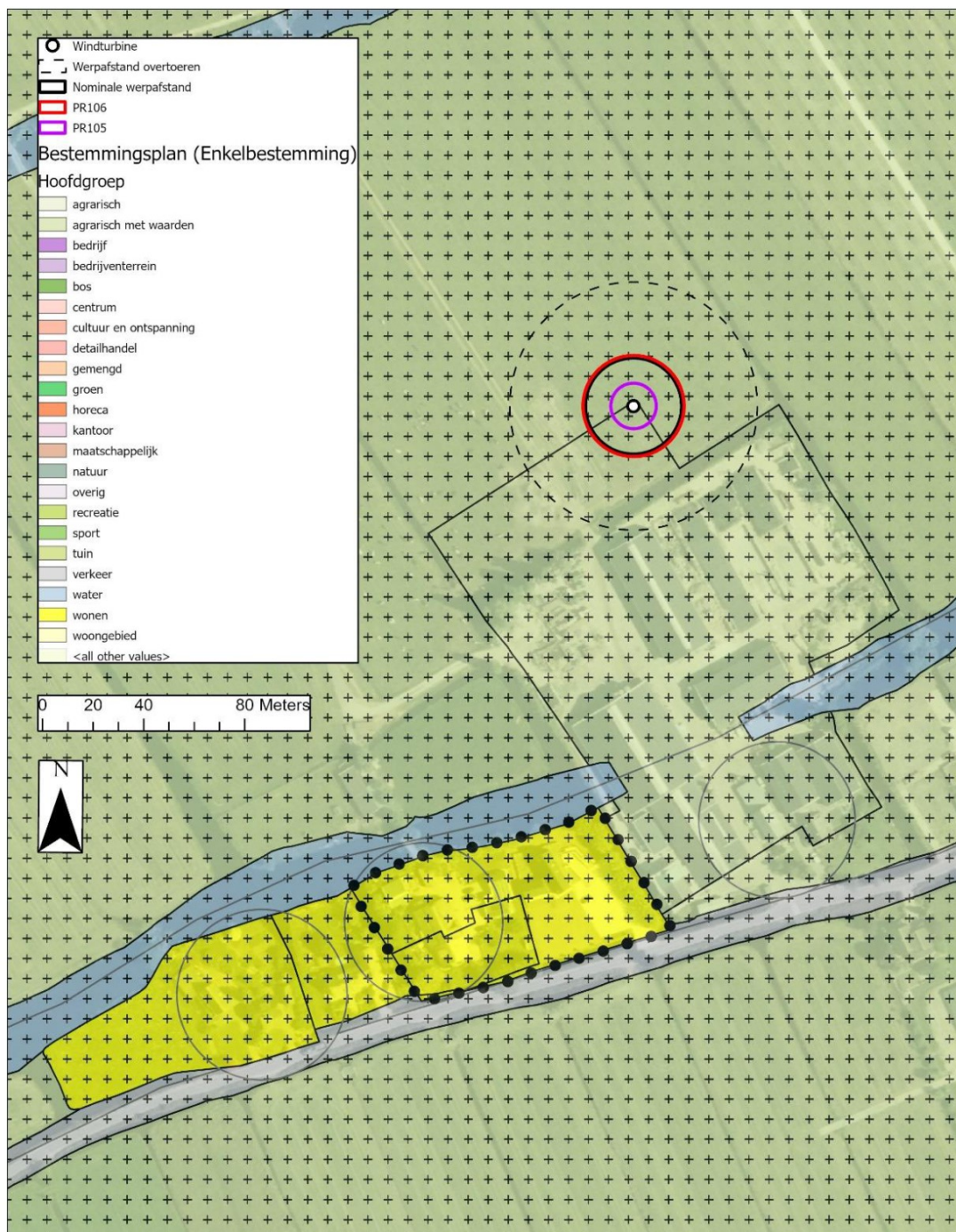
figuur 2: PR-contouren en werpafstanden van de voorgenomen windturbine. Binnen de 10^{-5} /jaar en 10^{-6} /jaar contour staan geen gebouwen. De gebouwen die net binnen de werpafstand bij overtoeren staan, behoren bij het bedrijf van de initiatiefnemer.
