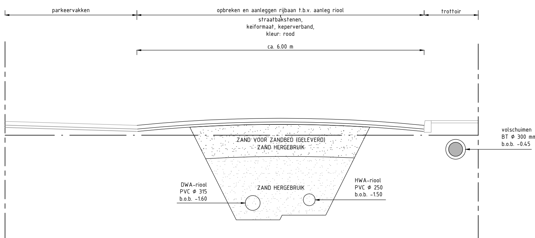
PRINCIPE PROFIEL KERKSTRAAT: VOLSCHUIMEN BESTAAND RIOOL EN AANBRENGEN TOEKOMSTIG RIOOL
